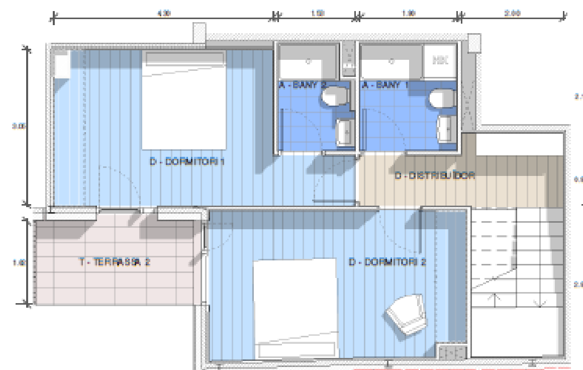
PLANTA PRIMERA
